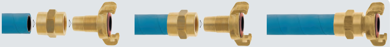
Einfache Montage ohne teures Einpresswerkzeug (Schraubenschlüssel genügt)
