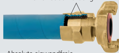
Einfache Montage ohne teures Einpresswerkzeug (Schraubenschlüssel genügt)
